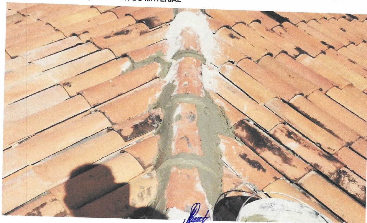
FOTO 20 - REVISÃO EM COBERTURA COM TELHA CERAMICA TIPO CANAL COMUM, ITABAIANA OU SIMILAR, COM REPOSIÇÃO DE 10% DO MATERIAL
